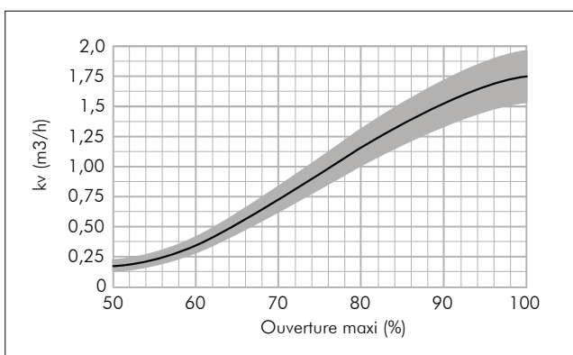
Kv vs. ouverture maxi moteur - primaire chauffage
