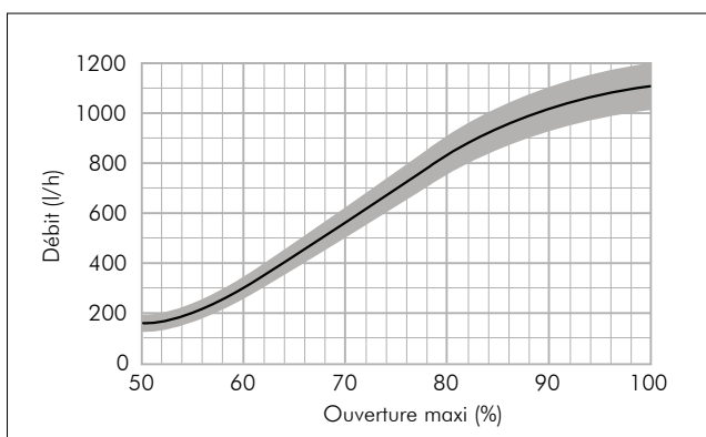
Débit vs. ouverture max. moteur - primaire ECS
